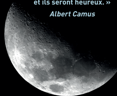
La Lune par Venus : © CNES, 2017
